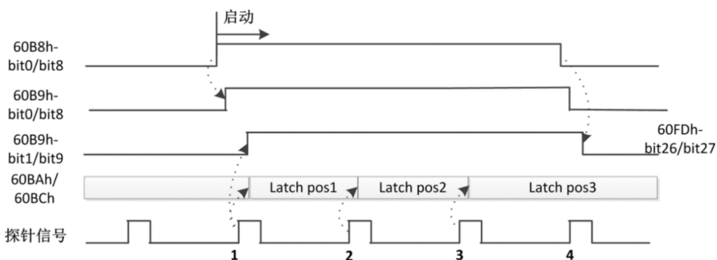
连续模式上升沿触发情况
