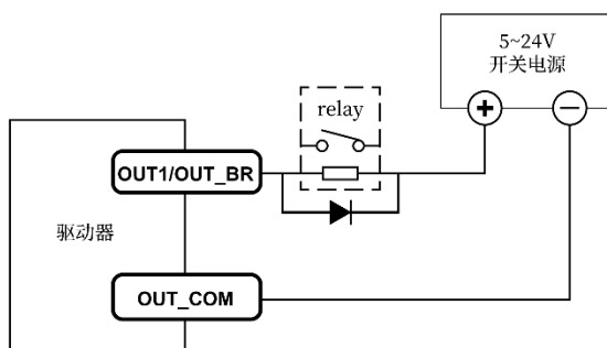
输出信号与继电器相连
