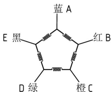
五相电机环形接线示意图
