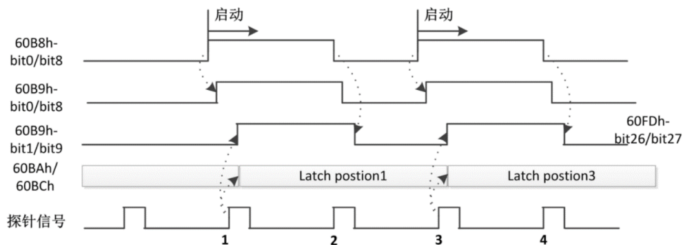
单次模式上升沿触发情况
