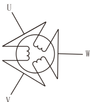
三相电机接线示意图
