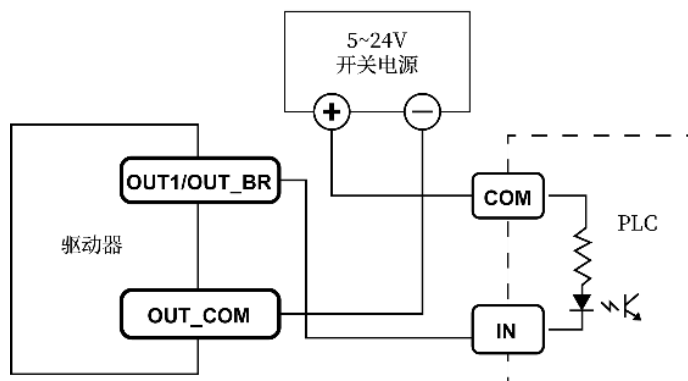
输出信号灌电流输出与 PLC 输入相连的连接方式
